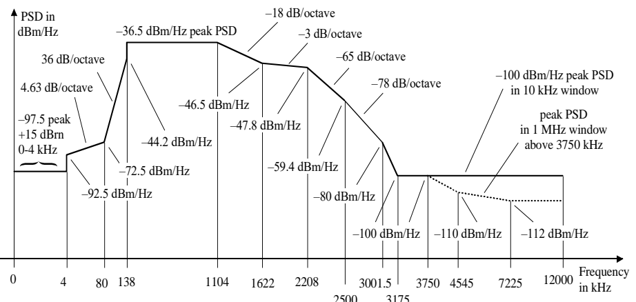
Figura 6 – Máscara de DEP para modems de central ADSL 2+ com espectro não sobreposto
