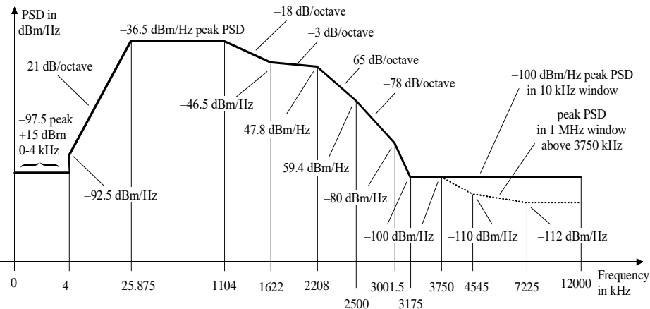
Figura 5 – Máscara de DEP para modems de central ADSL 2+ com espectro sobreposto
