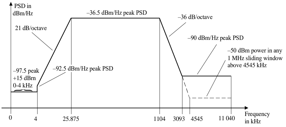
Figura 2 – Máscara de DEP para modems de central ADSL2 com espectro sobreposto
